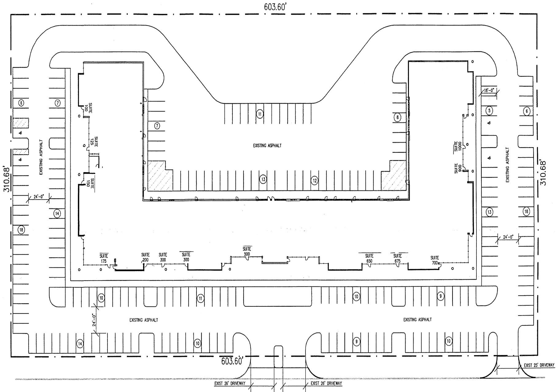
☉ SITE PLAN
